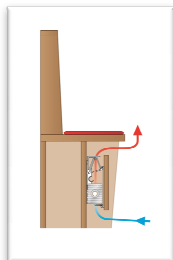
Kirchen Sitzbankbeheizung (technische Skizze): Heizleiste Classic von Variotherm
